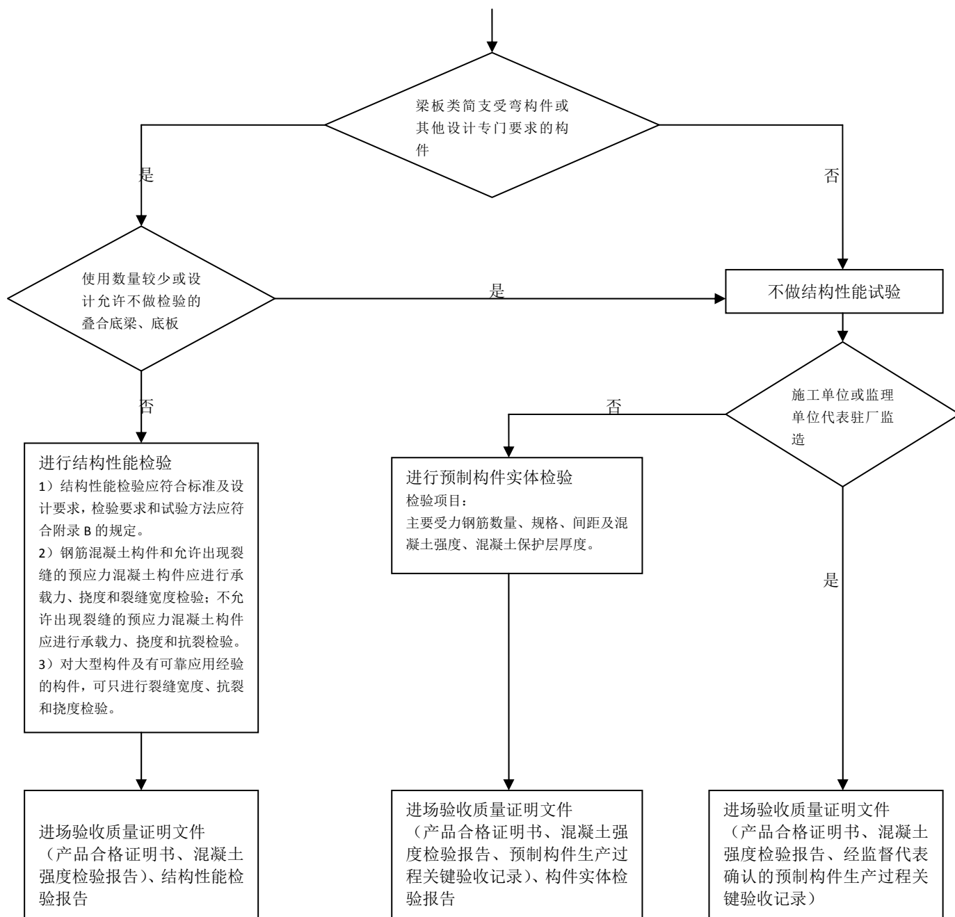
预制构件结构性能检验流程图
