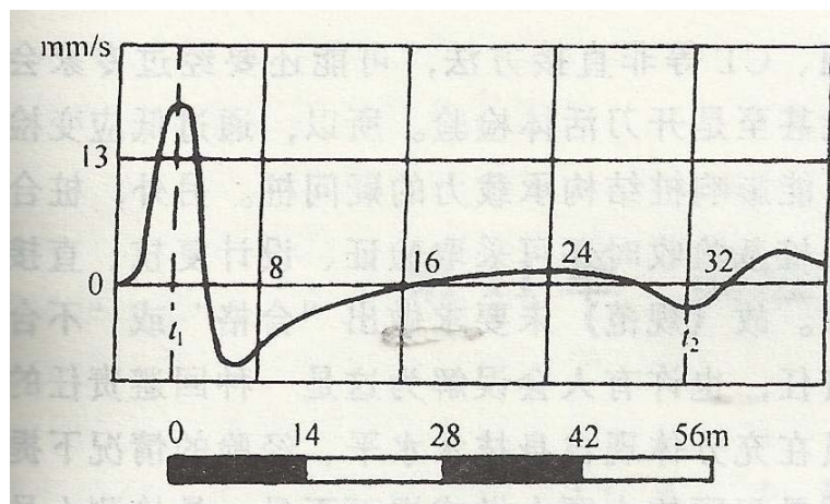
图：嵌岩桩实测波形
