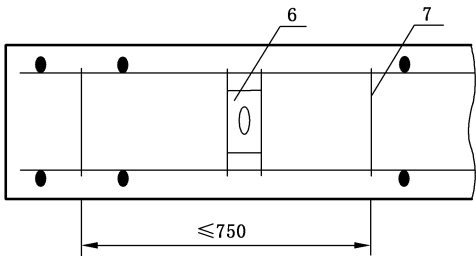
b) 网笼构造示意图
