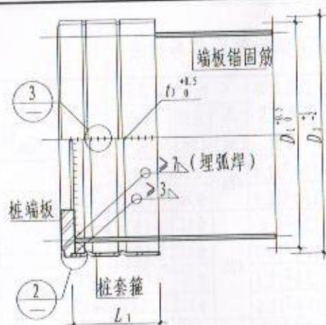
桩端板与套箍连接详图
