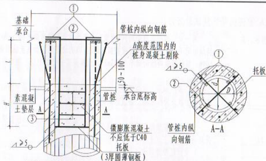
抗拔管桩与承台连接详图
