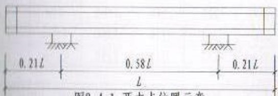
图8.4.1 两支点位置示意
