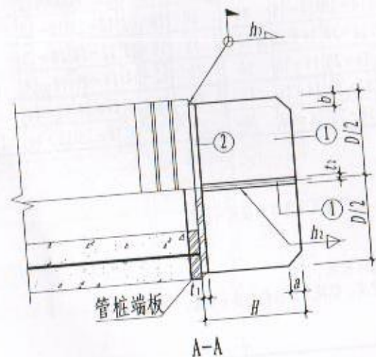
B型(平底十字形闭口)钢桩尖详图
