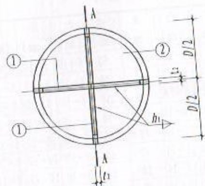
B型(平底十字形闭口)钢桩尖详图
