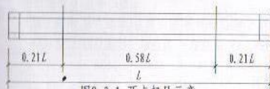
图8.3.1 两点起吊示意
