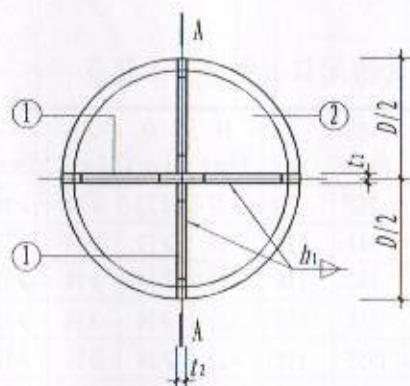
C型（尖底十字形闭口）钢桩尖详图
