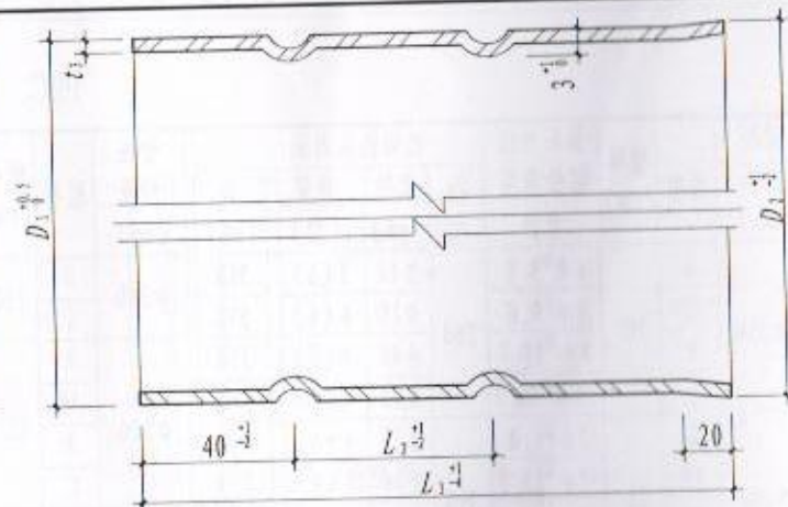
桩套箍剖面图
