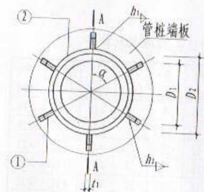
A型(开口形)钢桩尖详图
