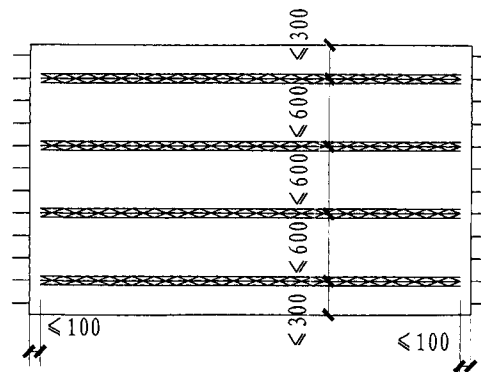
图4.8.1 钢筋桁架布置示意
