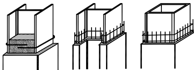
图 6-2 钢柱采用外包混凝土防护
