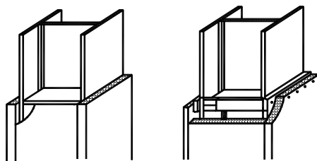
图 6-1 钢柱采用防火板防护
